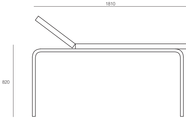
Tubular Frame
